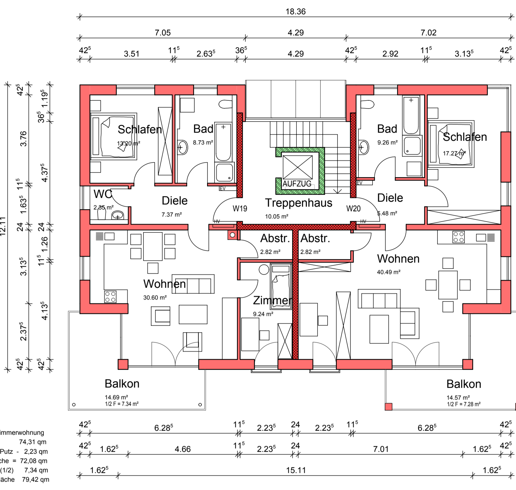
2. OBERGESCHOSS
