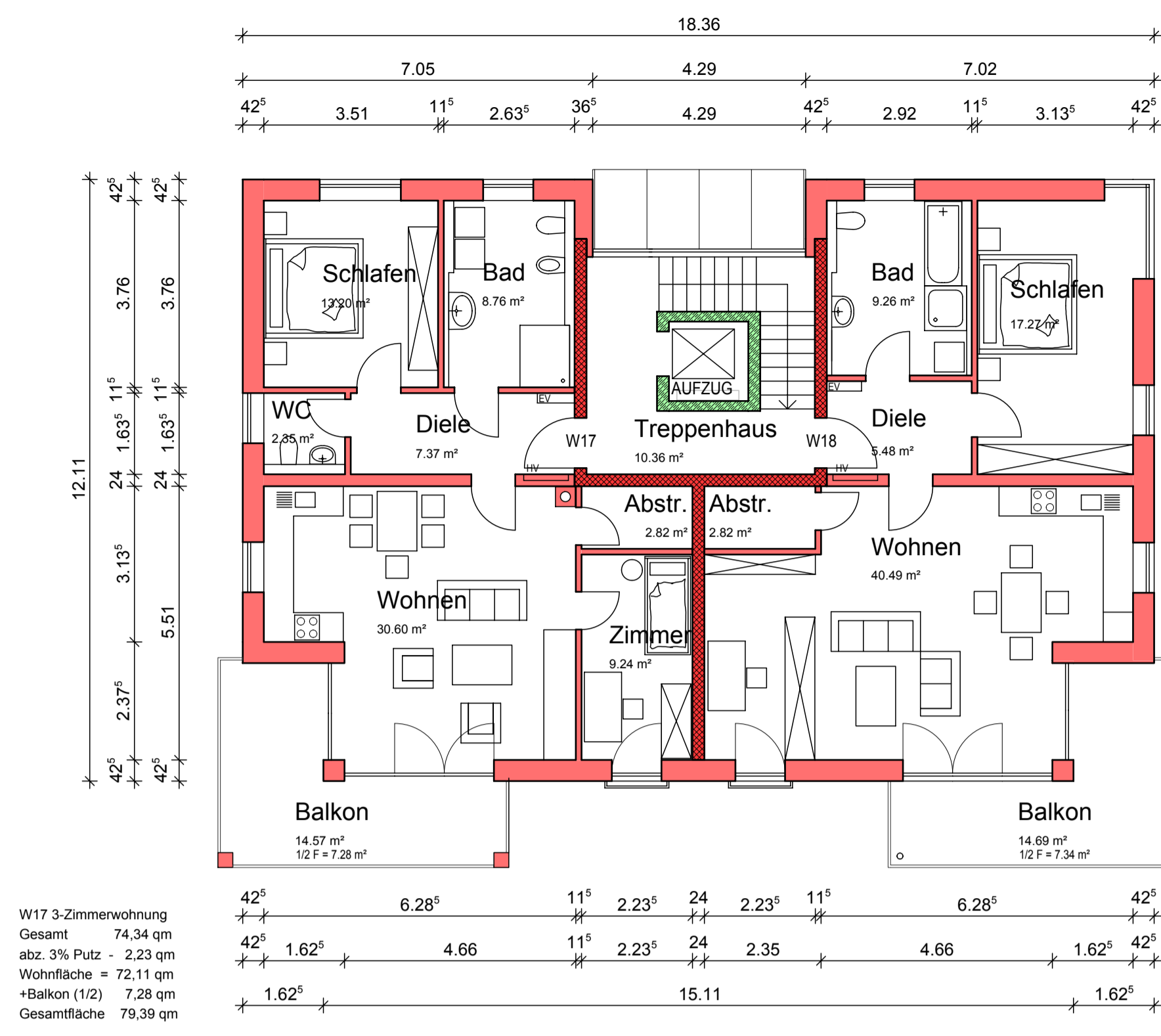
1. OBERGESCHOSS
