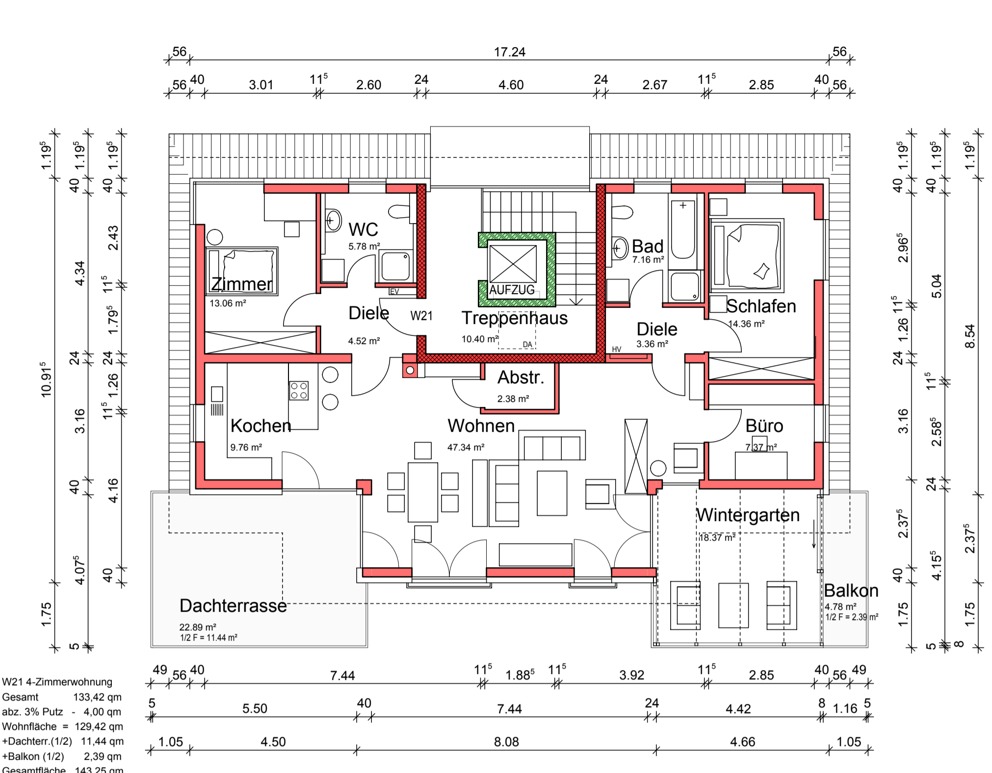
3. OBERGESCHOSS
